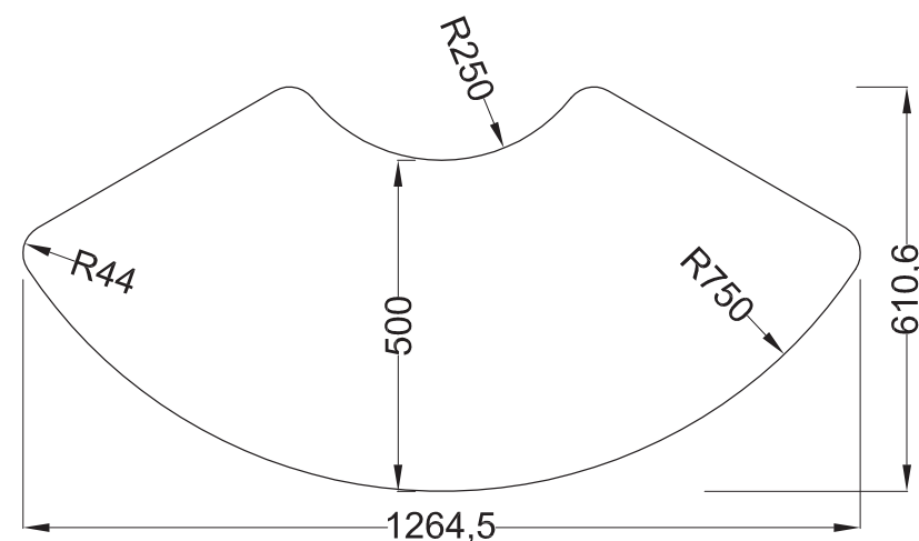
DIMENSIONI PIANO DI LAVORO TAVOLO ARCO IN MM. Dimension Table Arco in mm / Dimensions Table Arco in mm
